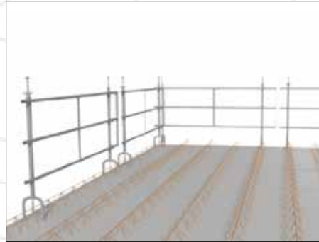
Filigrandecken-Geländer 1,50 m verzinkt, Gewicht 20,4 kg
